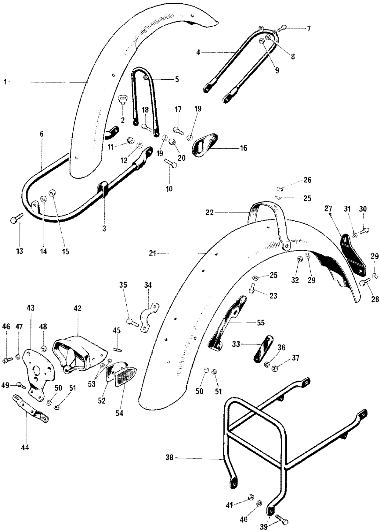
Fig. 27. MUDGUARDS (FENDERS)
