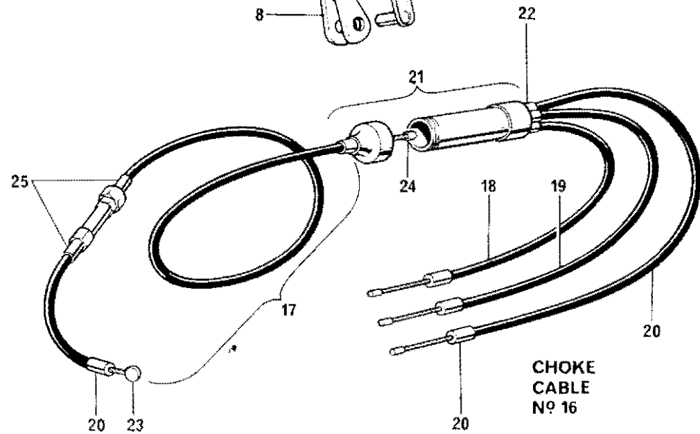
Fig. 29. CONTROL CABLES
