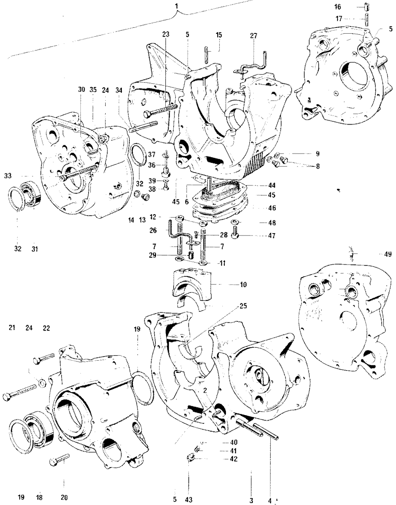
Fig. 2. CRANKCASES
