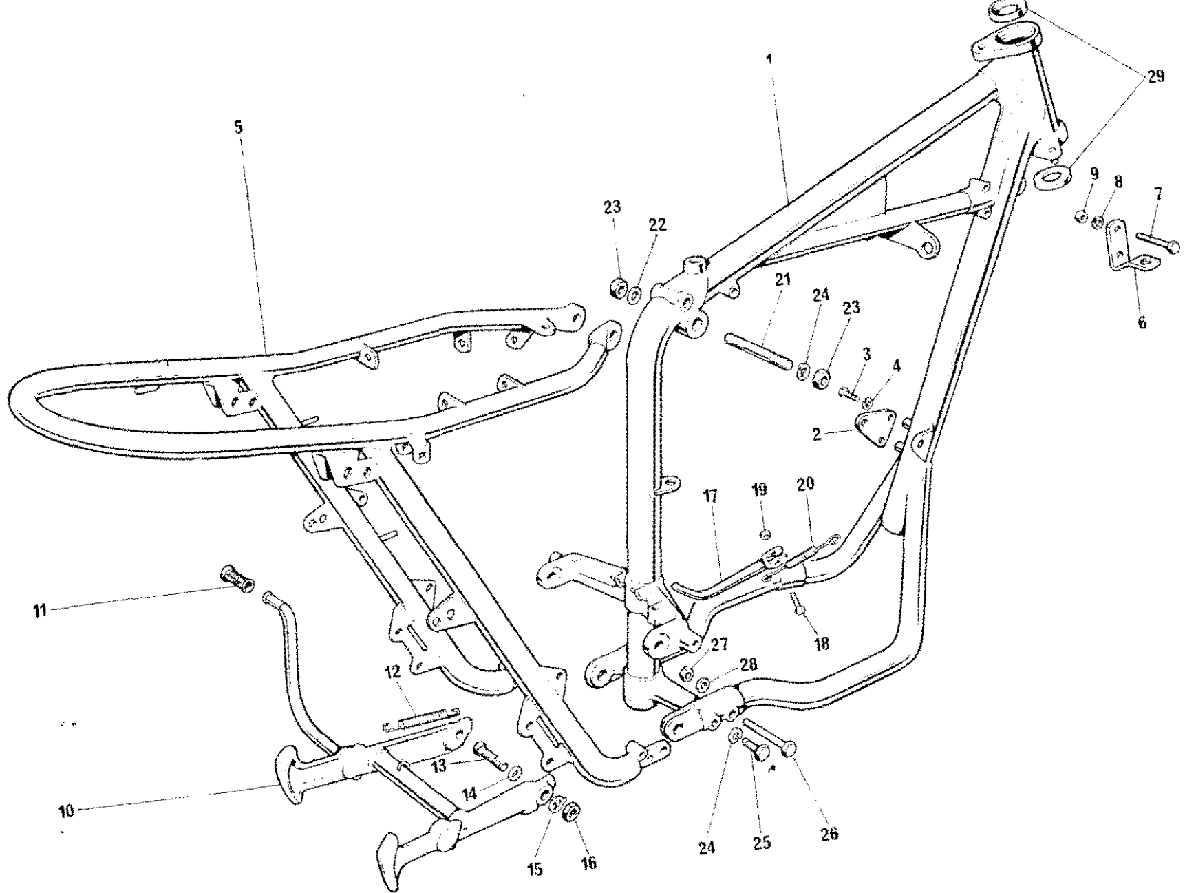
Fig. 14. FRAME
